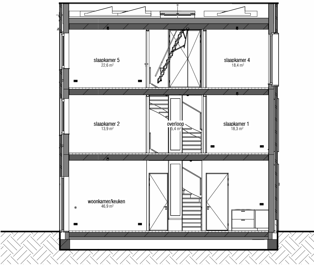
doorsnede 1:100
