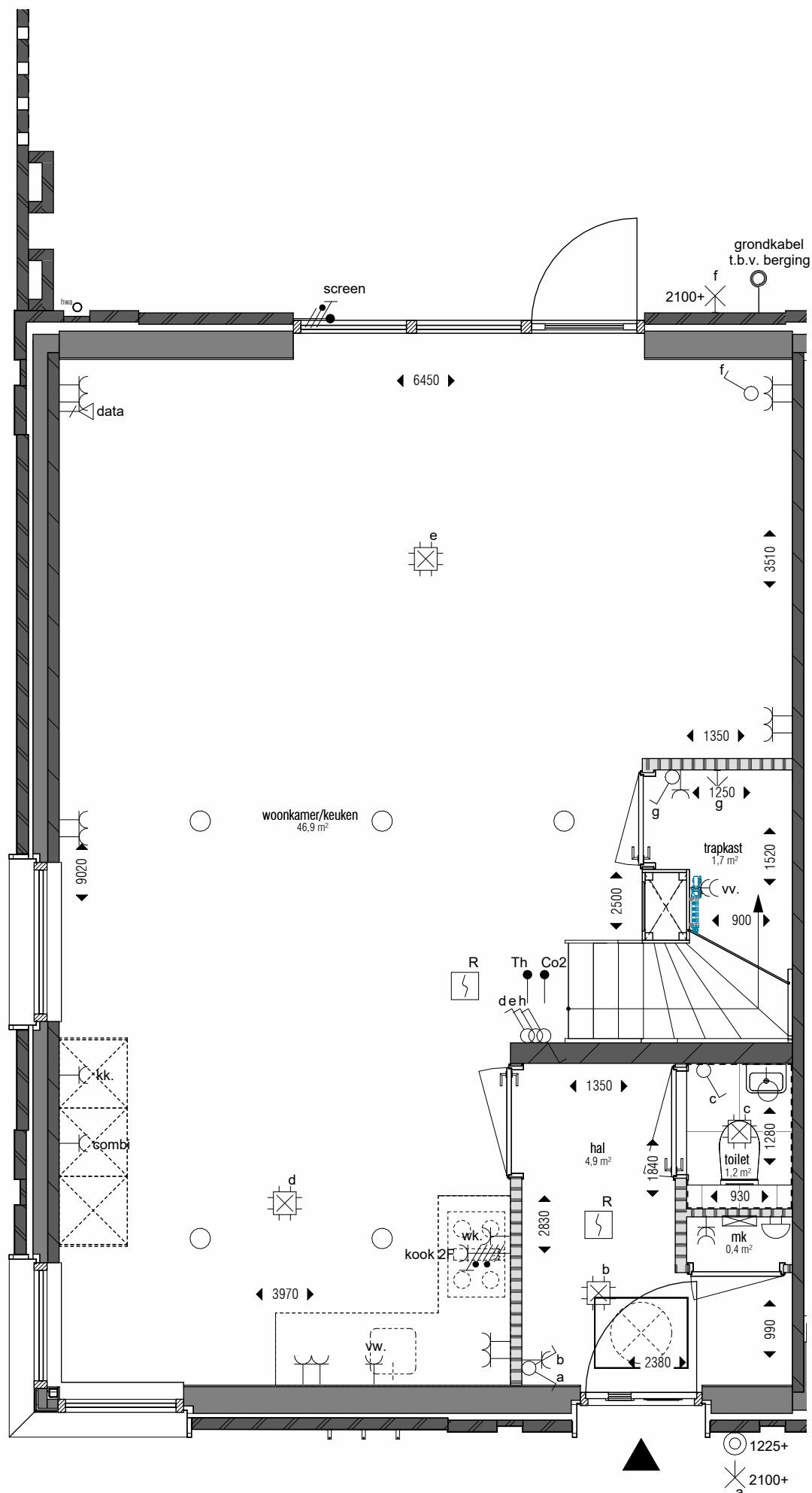
begane grond 1:50
