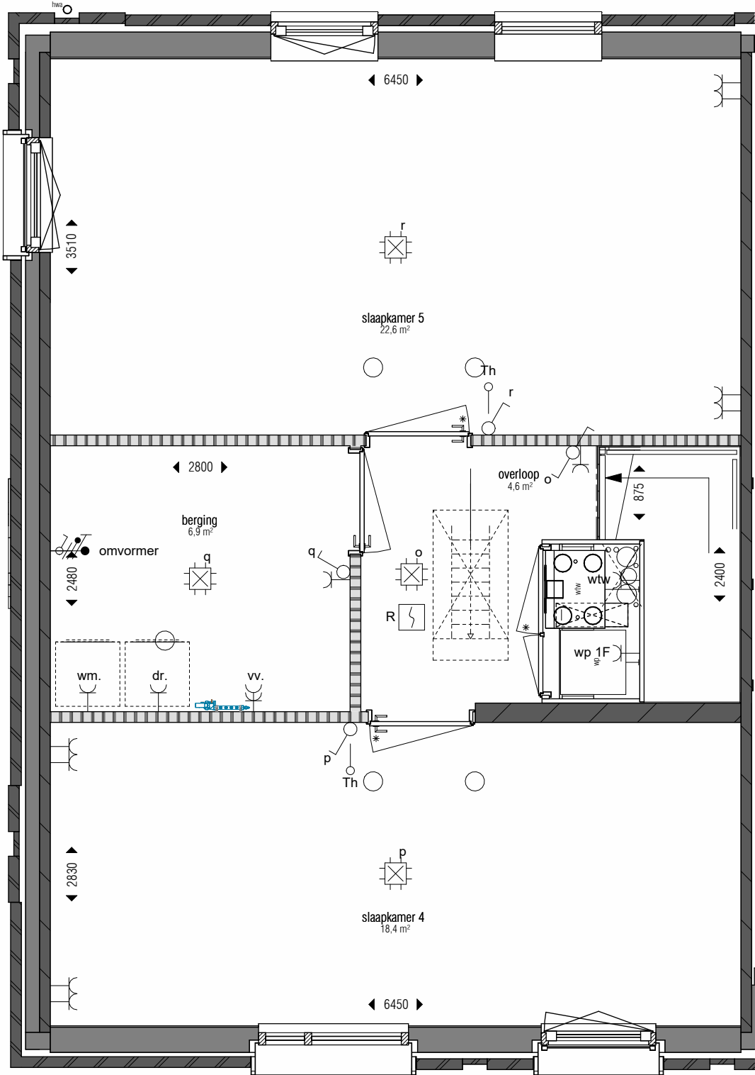
tweede verdieping 1:50
