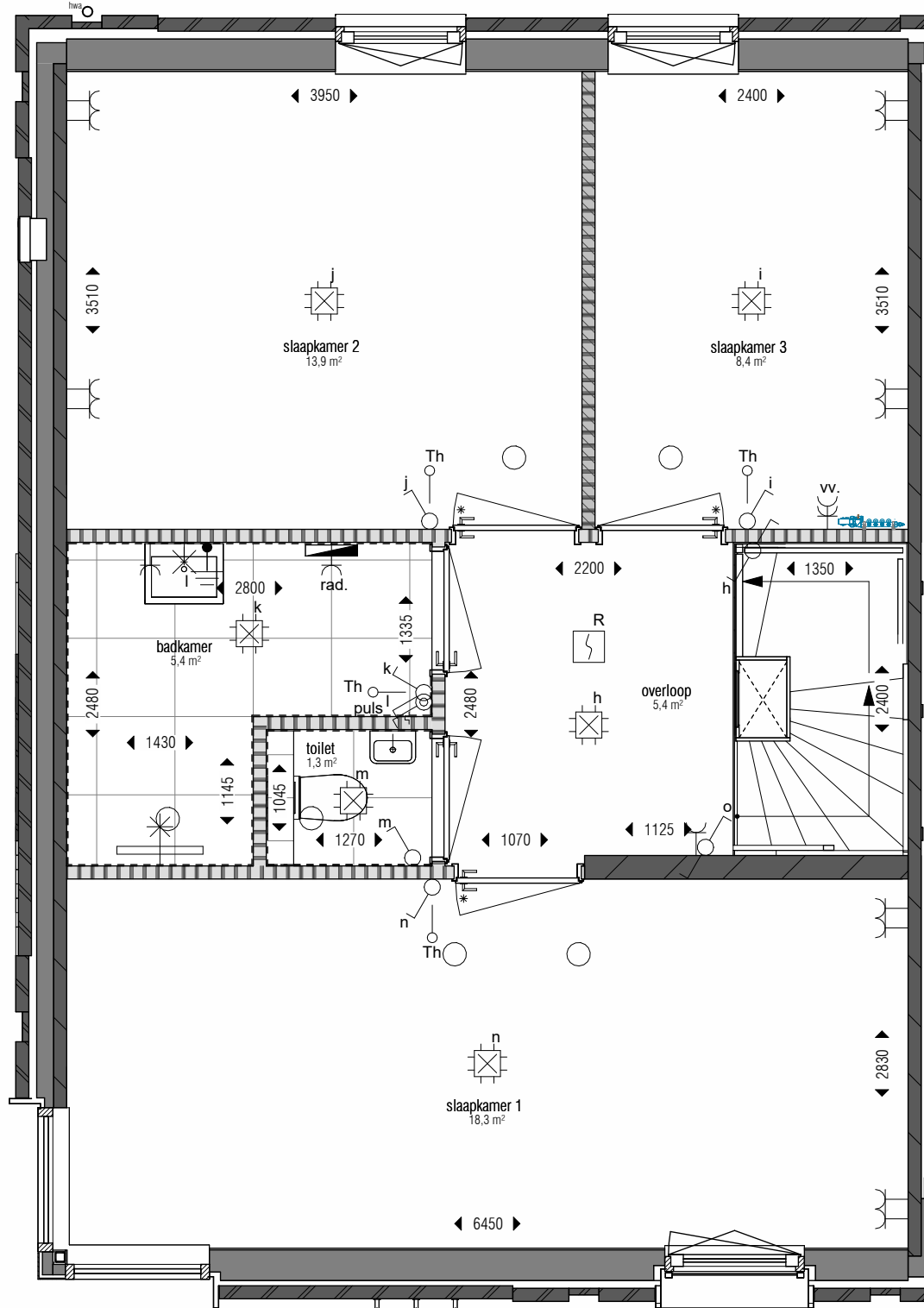
eerste verdieping 1:50
