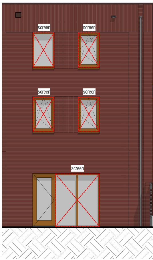
achtergevel 1:100
